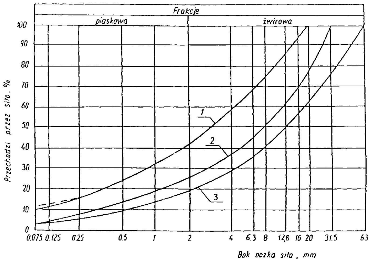
Rysunek 1. Pole dobrego uziarnienia kruszyw przeznaczonych na podbudowy wykonywane metodą mechaniczną.
